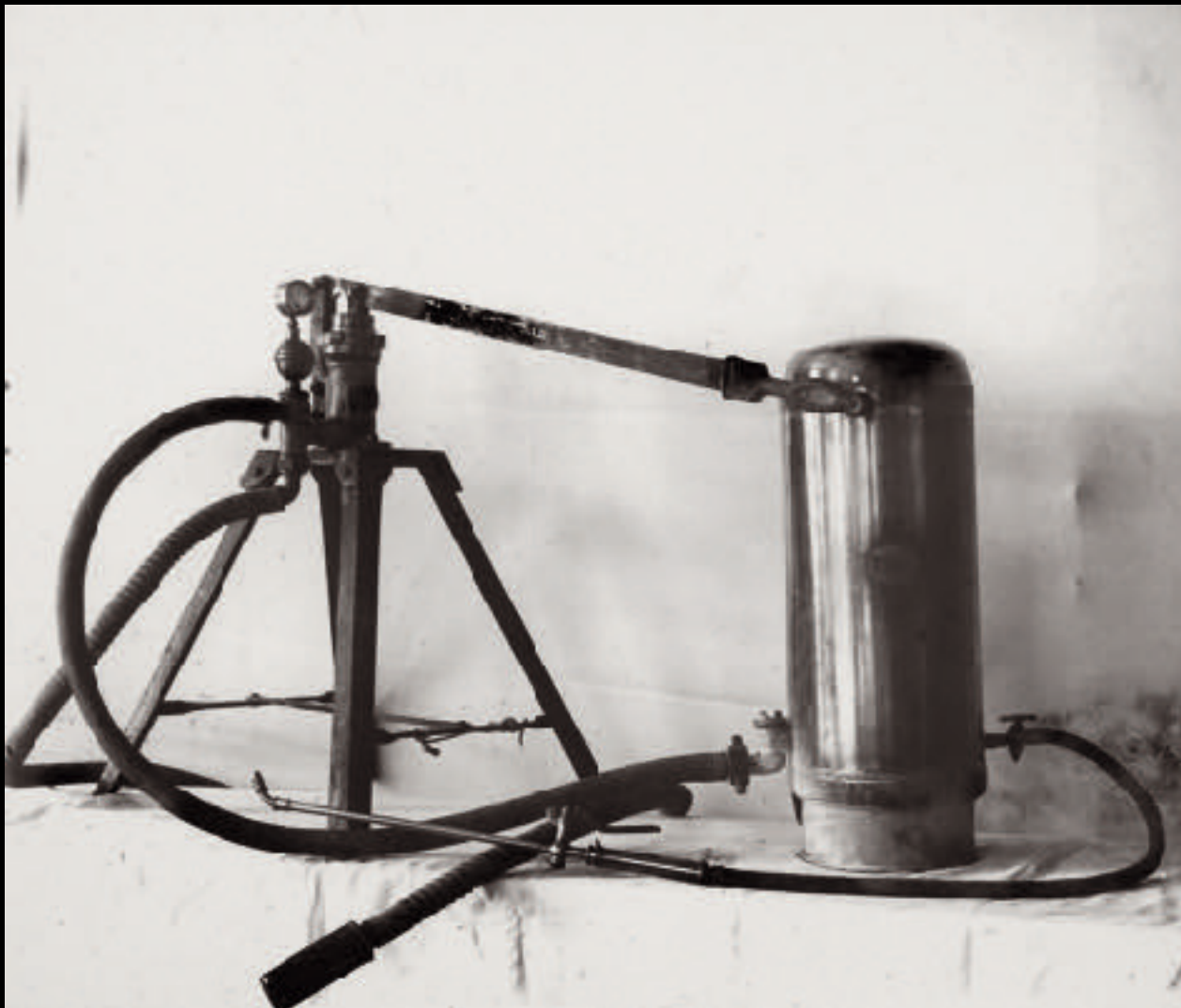
Pulvérisateur à pression avec pompe indépendante, système Nicolas
