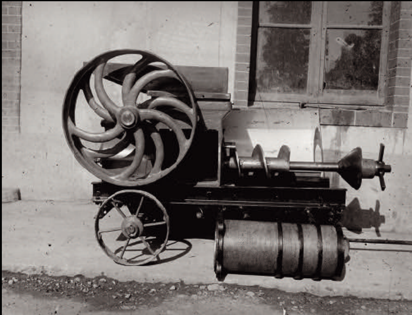
Pressoir continu Colin (ouvert)
